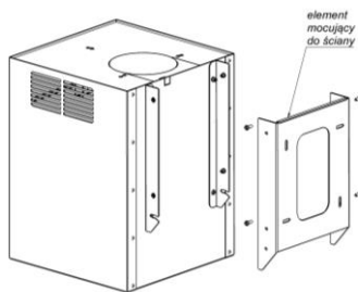
Rys. 8 Montaż okapu (w wersji przyściennej)
