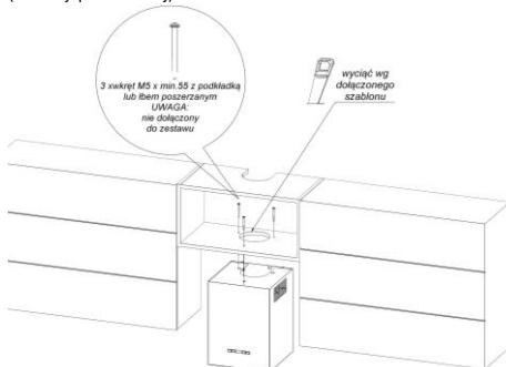
Rys. 10 Montaż okapu (w wersji poszafkowej)
