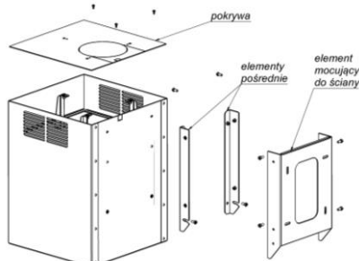
Rys. 9 Demontaż mocowania przyściennego
