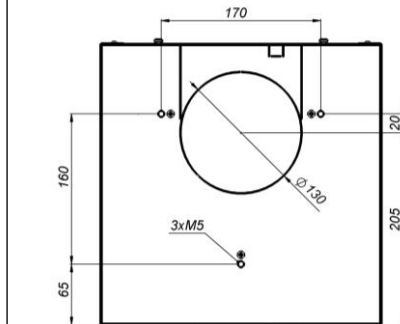
Rys. 3 wymiary otworów montażowych u góry okapu
