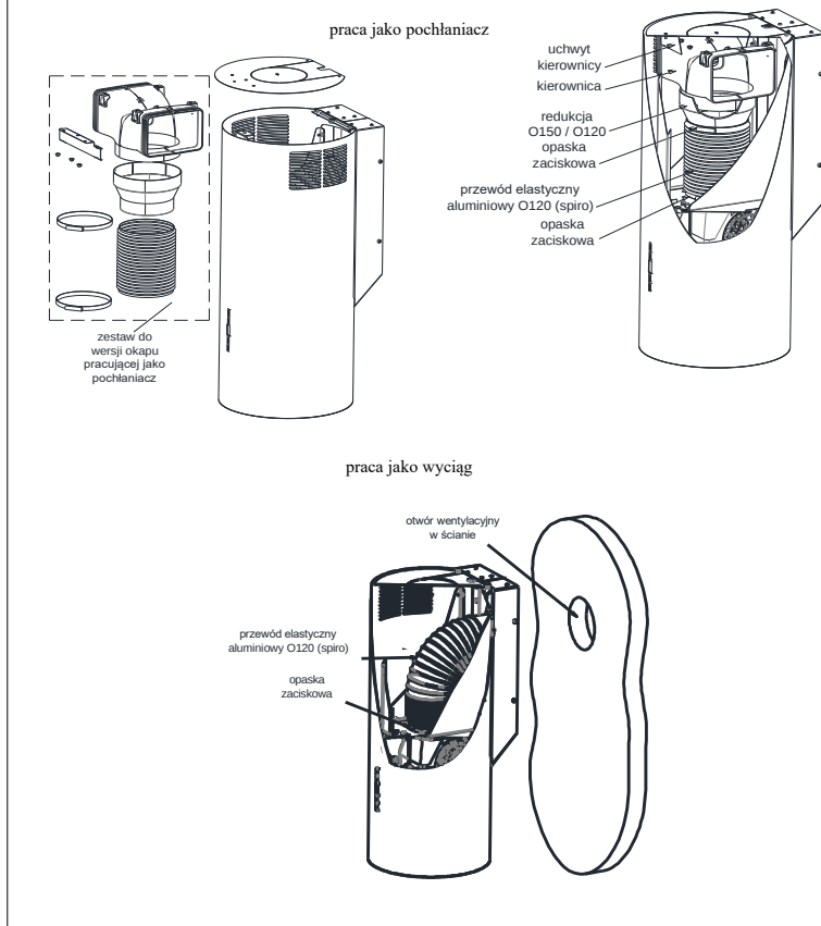
Rys. 3 Opcje montażu: pochłaniacz lub wyciąg
