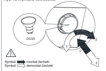
Rys. 13 Wymiana oświetlenia.
