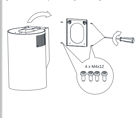
Rys. 10 Montaż okapu na uchwyty ścienny.
