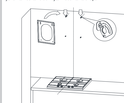
Rys. 10 Montaż okapu na uchwyty ścienny.
